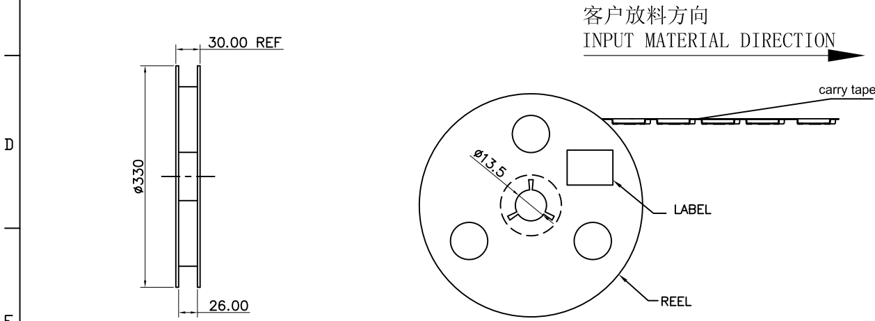
PH92-9B20C41A & 包装示意图
