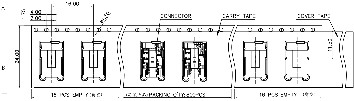
PH92-9B20C41A & 包装示意图
